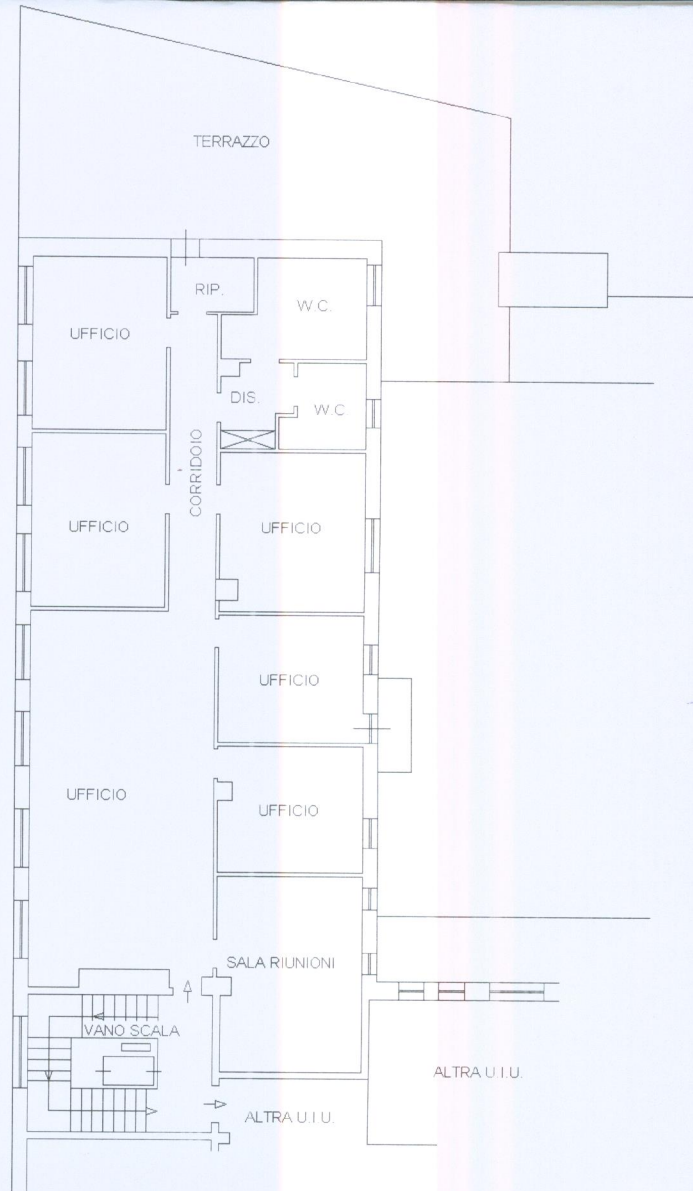
PIANO SECONDO H. 3,00
